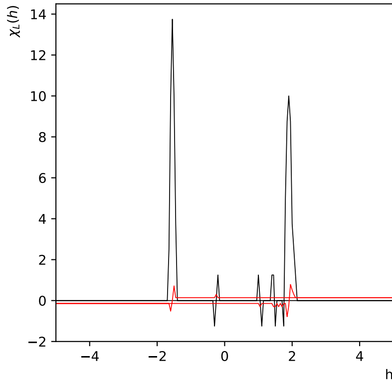
\chi_L(h) réseau de taille L=4 à T=1.5
