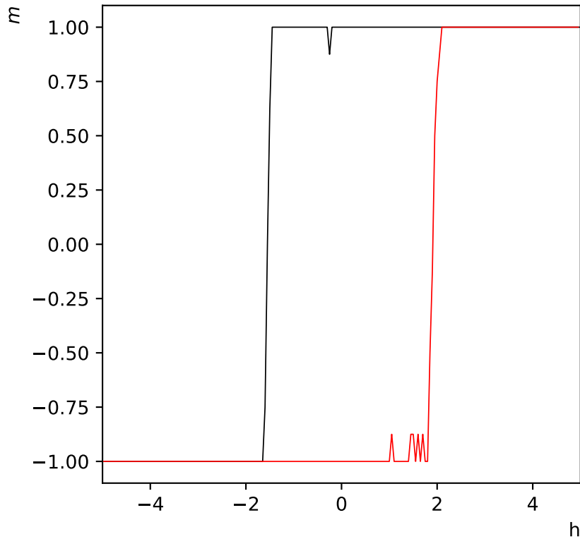
Hystérésis de l'aimantation réseau de taille L=4 - h=5 à T=1.5
